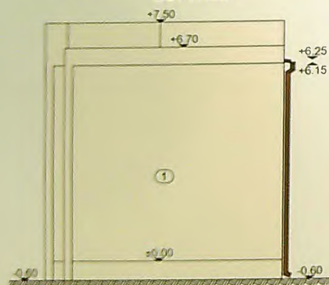
FAȚADĂ POSTERIOARĂ SC. 1:100
