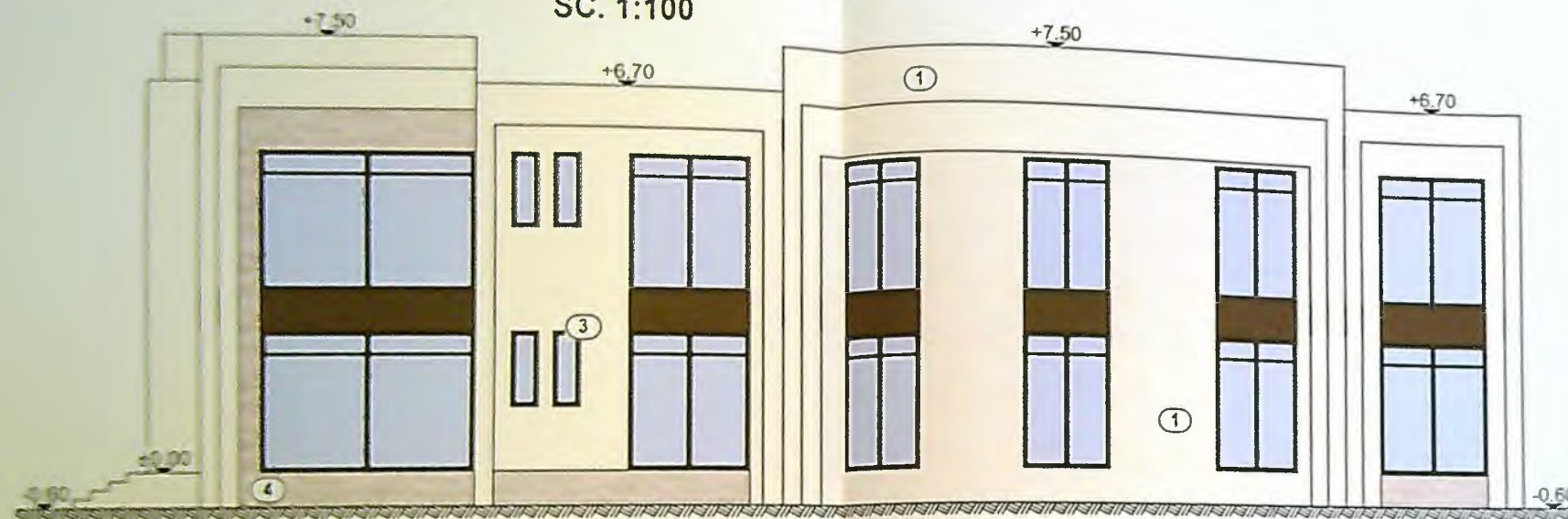
FAȚADĂ POSTERIOARĂ SC. 1:100
