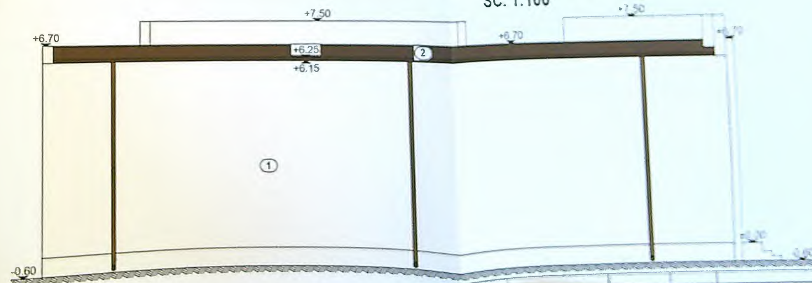
FAȚADĂ LAT.-STÂNGĂ SC. 1:100
