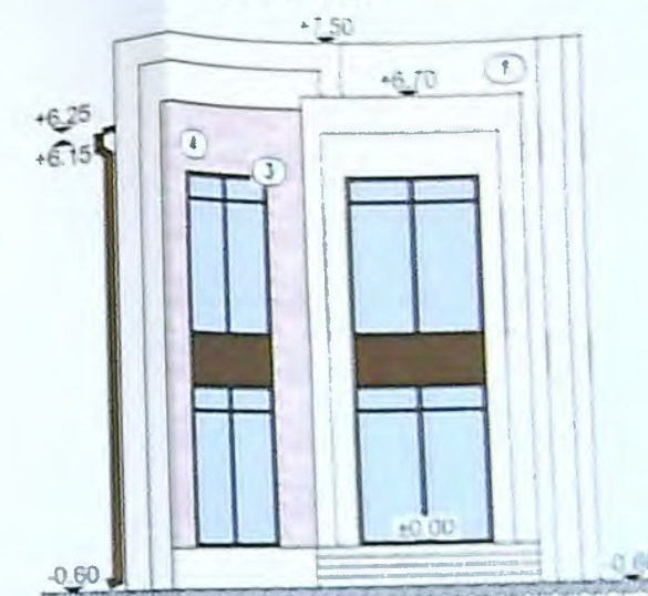
FAȚADĂ PRINCIPALĂ SC. 1:100
